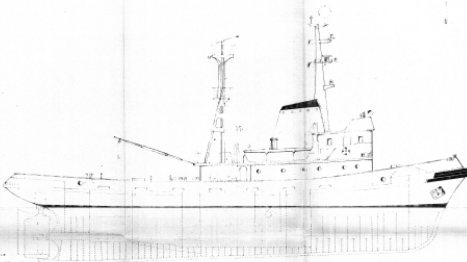
PROFILLO LONGITUDINALE
